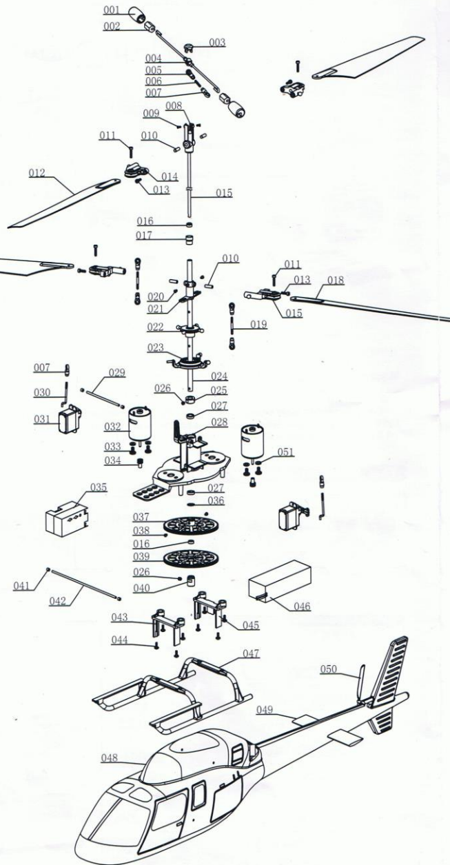
机体炸散图
